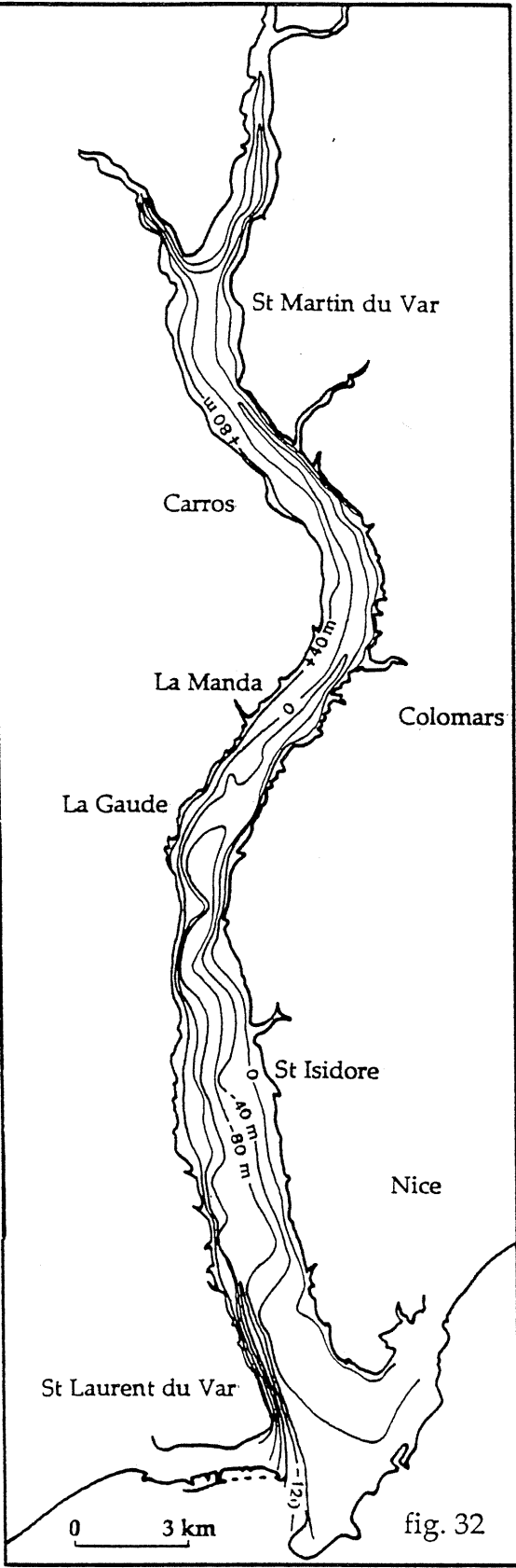
Fig. 32: Topographie du substratum des alluvions.
