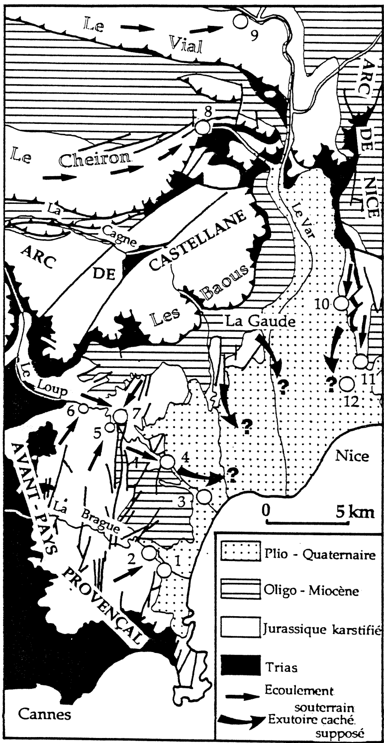
Fig. 14 : Principales sources et pertes karstiques situées au voisinage de la vallée du Var: 1 - sources Romaines ; 2 - sources de Biot ; 3 - sources des Tines ; 4 - perte du Loup ; 5 - source Merle ; 6 - source des Noyers ; 7 - source du Lauron ; 8 - source des Fontaniers ; 9 - source de La Mescla ; 10 - source temporaire de la Fuont-Santa ; 11 - source des Mourailles ; 12 - la Fontaine du Temple.
